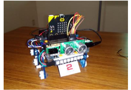
6足昆虫型ロボットの製作
